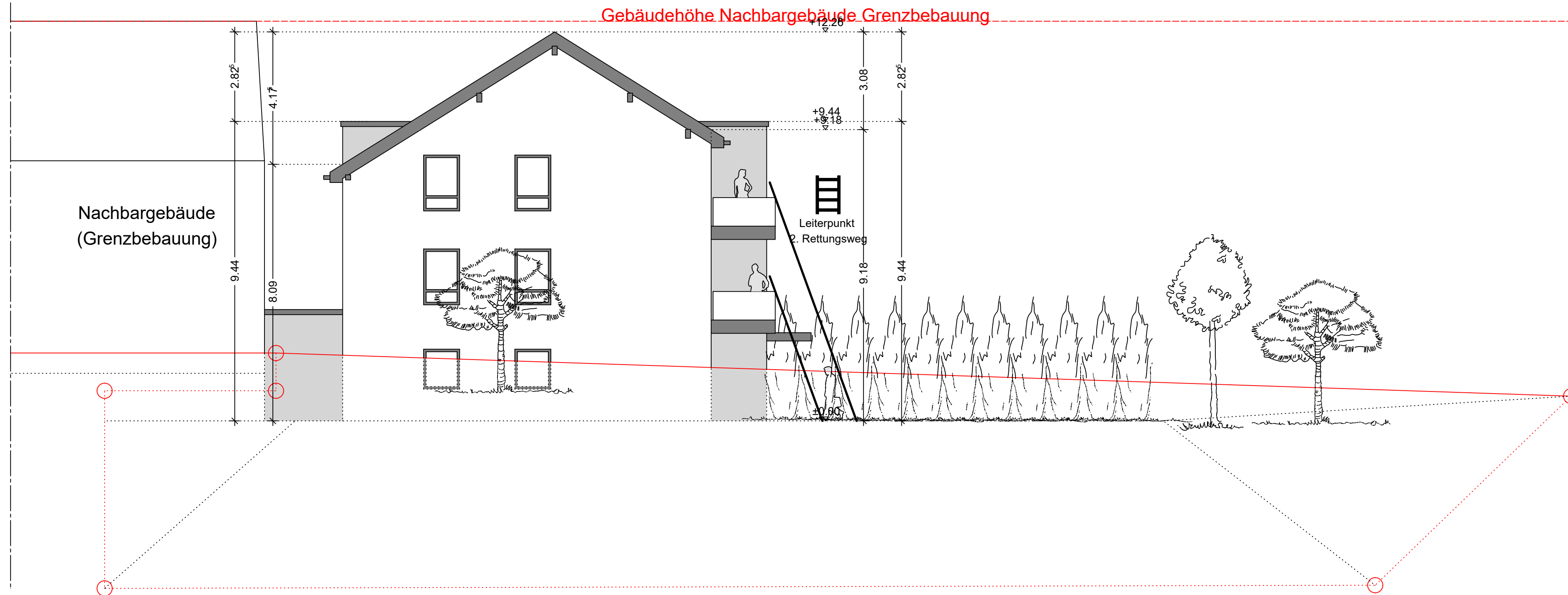
Ansicht Nord-Ost
