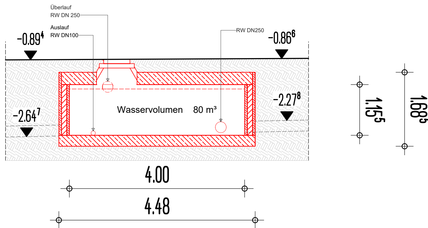
Schnitt A-A M1:50
