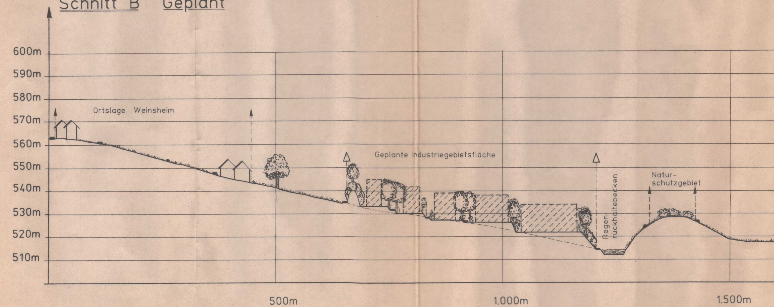
Schnitt B Geplant
