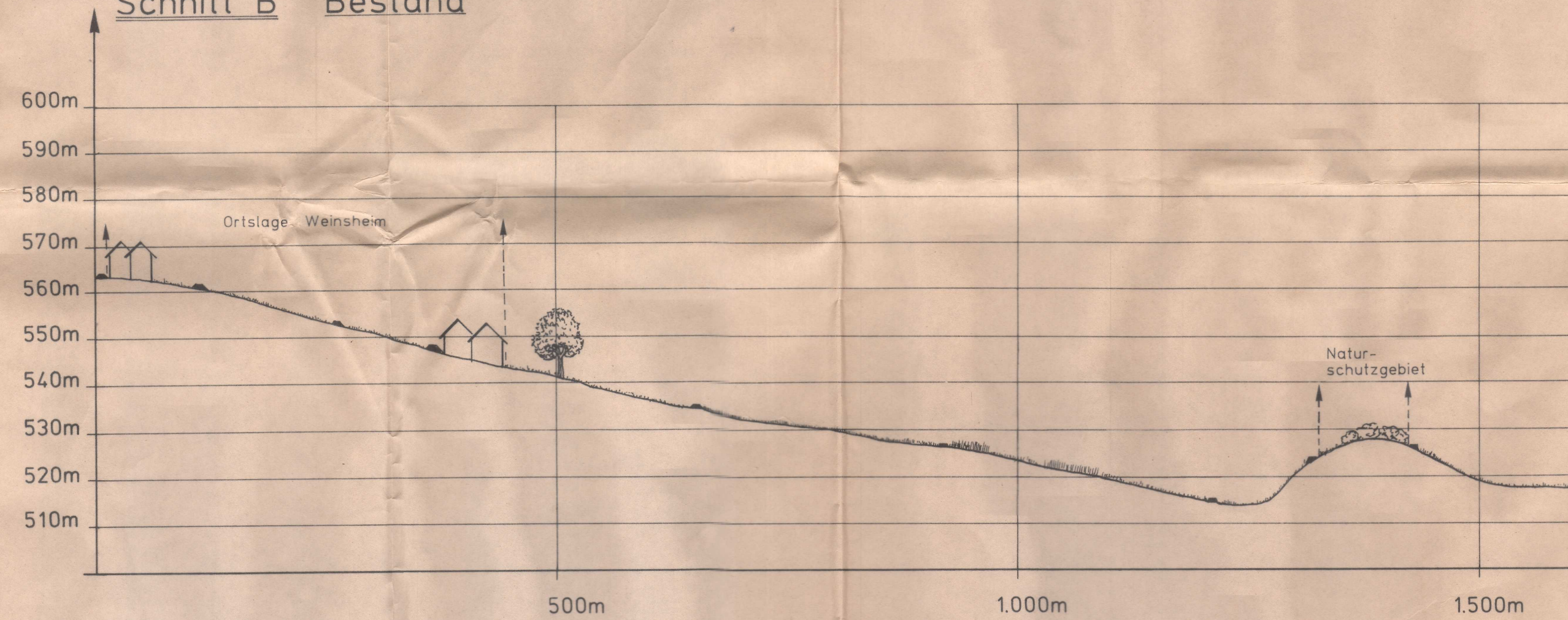
Schnitt B Bestand
